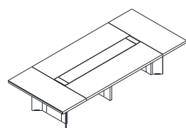
Ш3400xГ1500xВ750 мм
