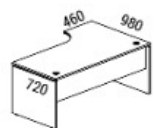
Стол эргономичный левый/правый
